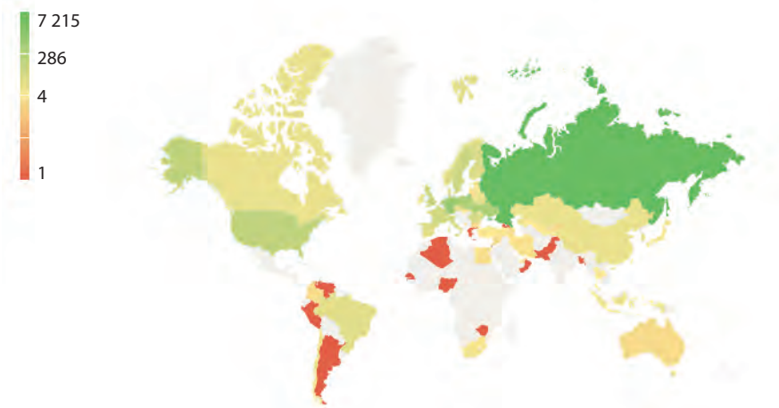
График 3. Географическая характеристика посещаемости сайта
